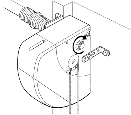
Abbildung 2: Öffnungsbewegung mit umgekehrtem Drehsinn des Antriebs
